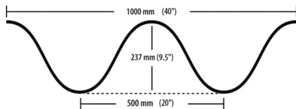
1 pav. Konstrukcijos lakšto banguotas profilis
