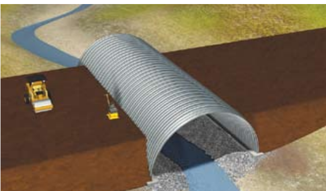
Konstrukcijos užpylimas sluoksniais
